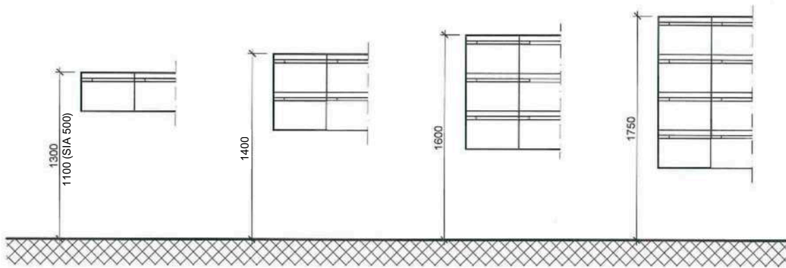
Aufputz-Montage
