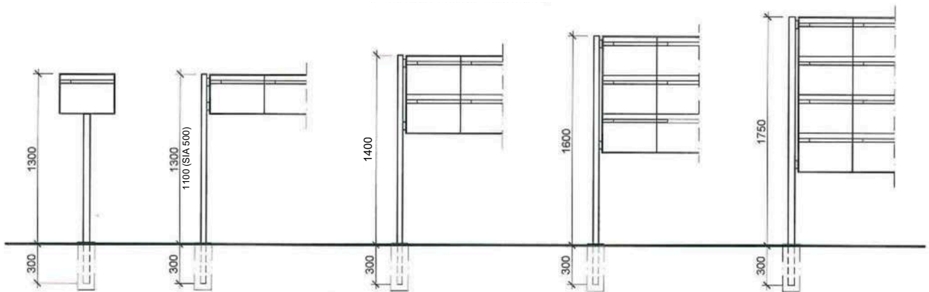
Freistehende Montage
